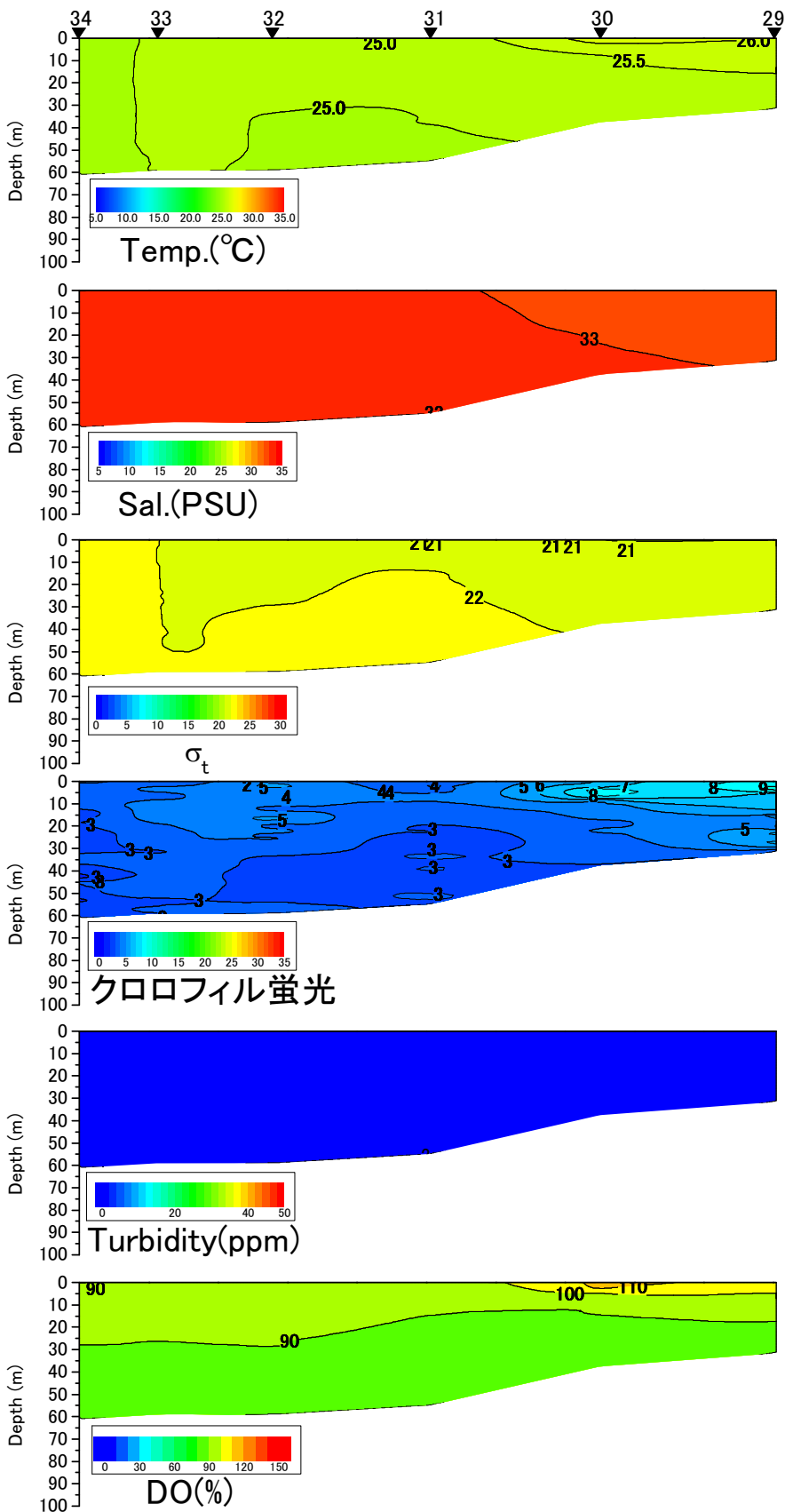
八代海西ラインの水温(°C)、塩分、密度( \sigma_t )、クロロフィル蛍光強度、濁度、溶存酸素飽和度(DO%)の鉛直面図(国土交通省の調査による) (2014年8月28日)
